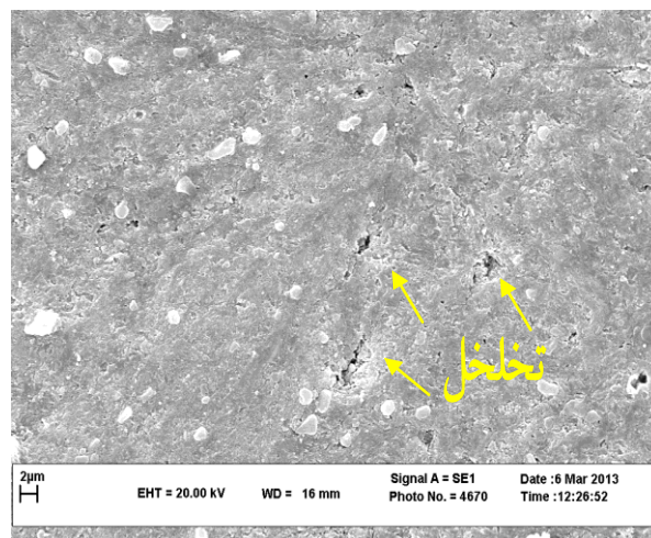
شکل ۵- تصویر SEM تهیه شده از نمونه حاوی ۱۰ درصد
