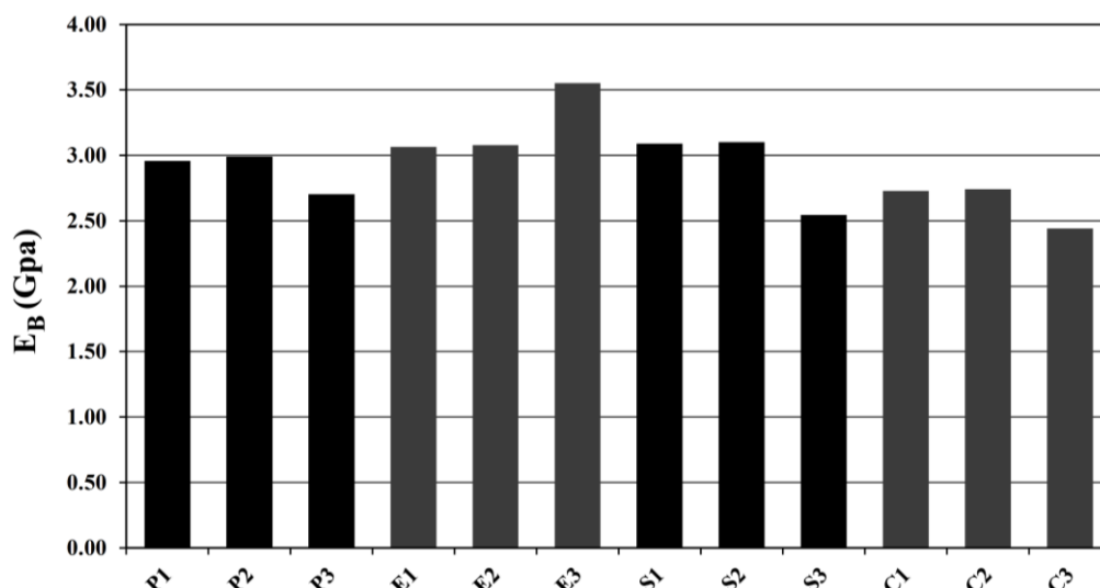
شکل ۴- مقادیر مدول کشسان مُماسی نمونه‌های خالص و کامپوزیتی
